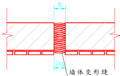
图 4.0.6 变形缝两侧排砖示意
