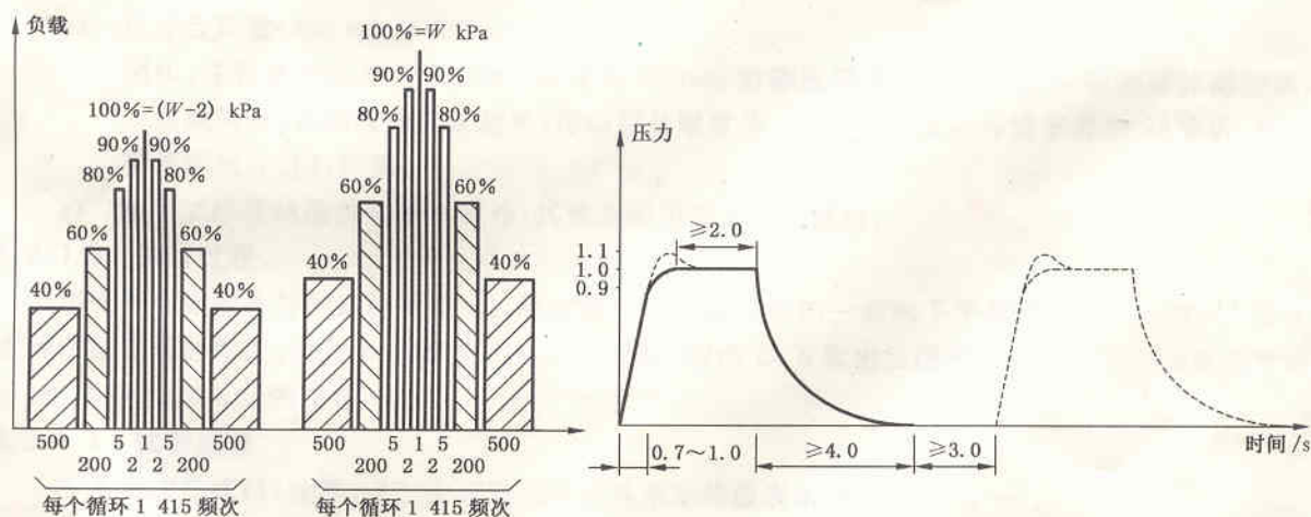
图 A.1 加压过程和压力脉冲示意图
