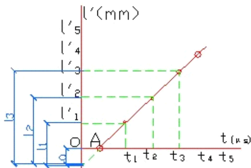
图 5.2.1-1 平测“时-距”图
