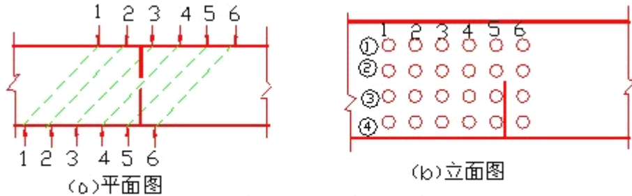
图 5.3.1 斜测裂缝测点布置示意图
