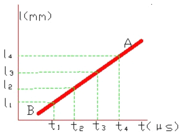
图 A.0.2 测空气声速的“时-距”图
