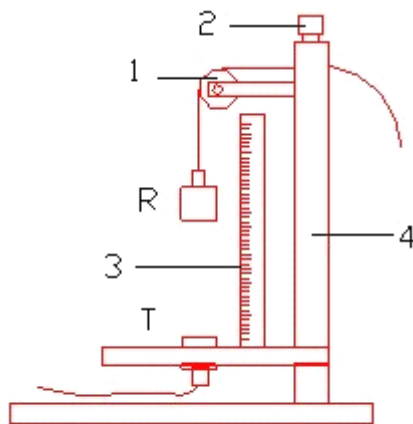
1-定滑轮 2-螺栓 3-刻度尺 4-支架
