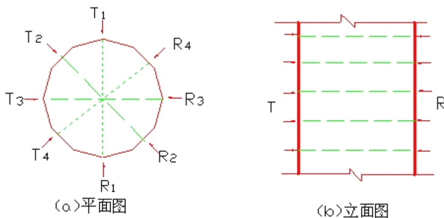
图 10.2.1 钢管混凝土检测示意图
