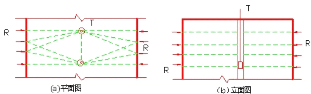
图 6.2.1-3 钻孔法示意图
