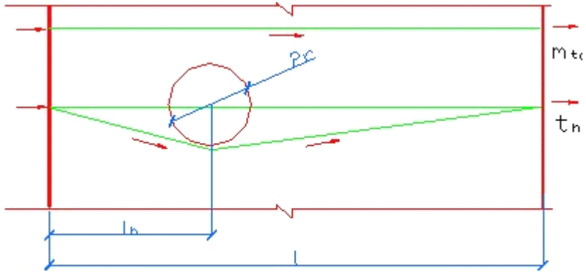
图 C.0.1 空洞尺寸估算原理图
