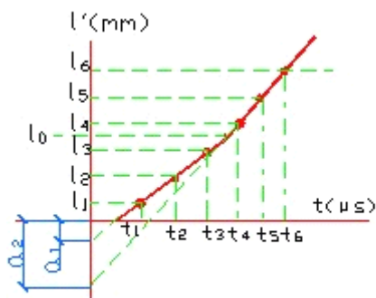
图 8.3.1 损伤层检测“时-距”图
