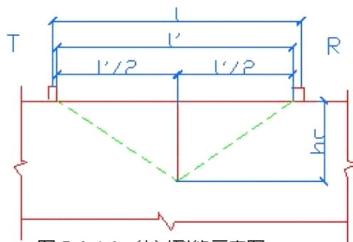
图 5.2.1-2 绕过裂缝示意图
