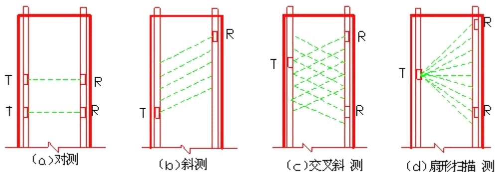
图 9.4.2 灌注桩超声测试方法剖面示意图
