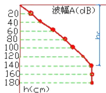
图 5.4.6 h-A坐标图
