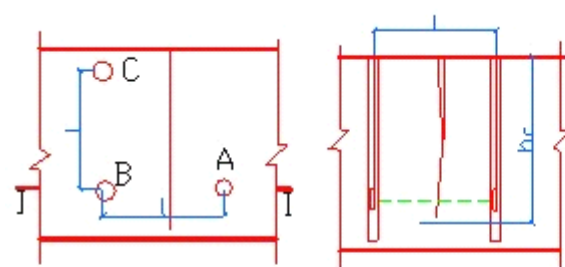
(a)平面图 C为比较孔
