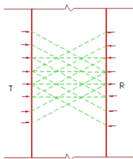
图 6.2.1-2 斜测法立面图
