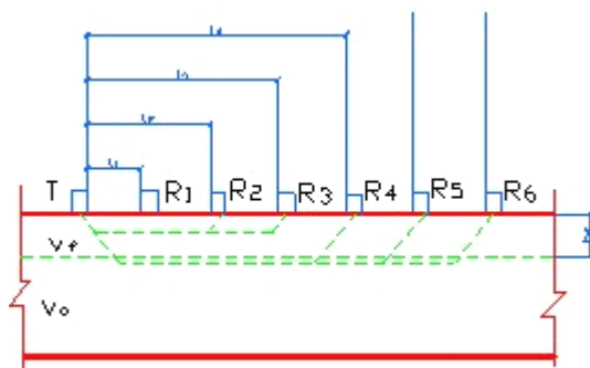
图 8.2.2 检测损伤层厚度示意图
